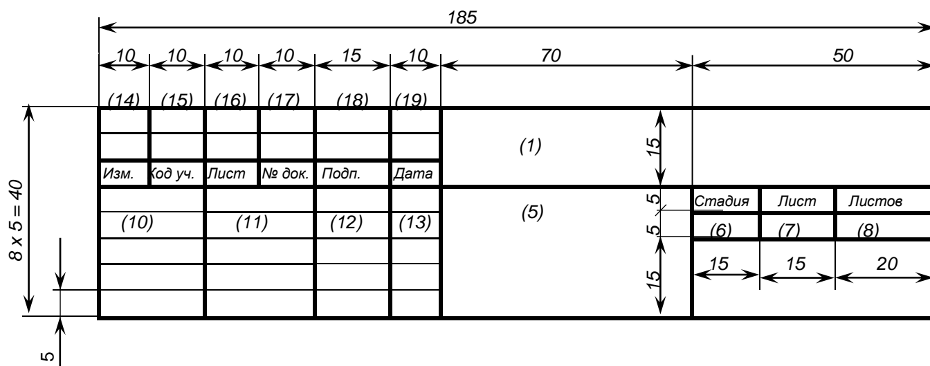
Рисунок Т.6 — Основная надпись и дополнительные графы к ней для всех видов текстовых документов (первые листы) по ГОСТ Р 21.1101, форма 5
