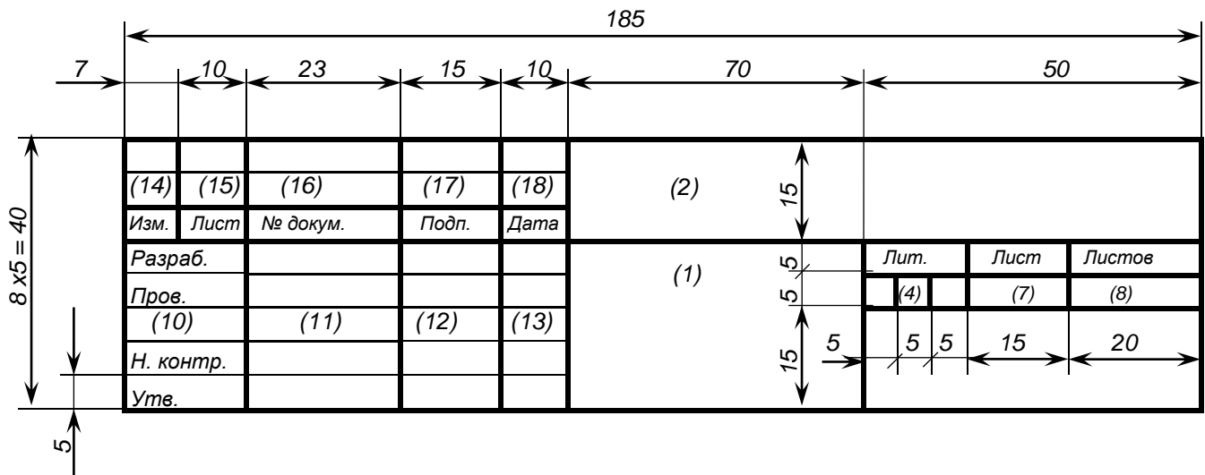
Рисунок Т.2 — Основная надпись для текстовых конструкторских документов (первый лист) по ГОСТ 2.104, форма 2
