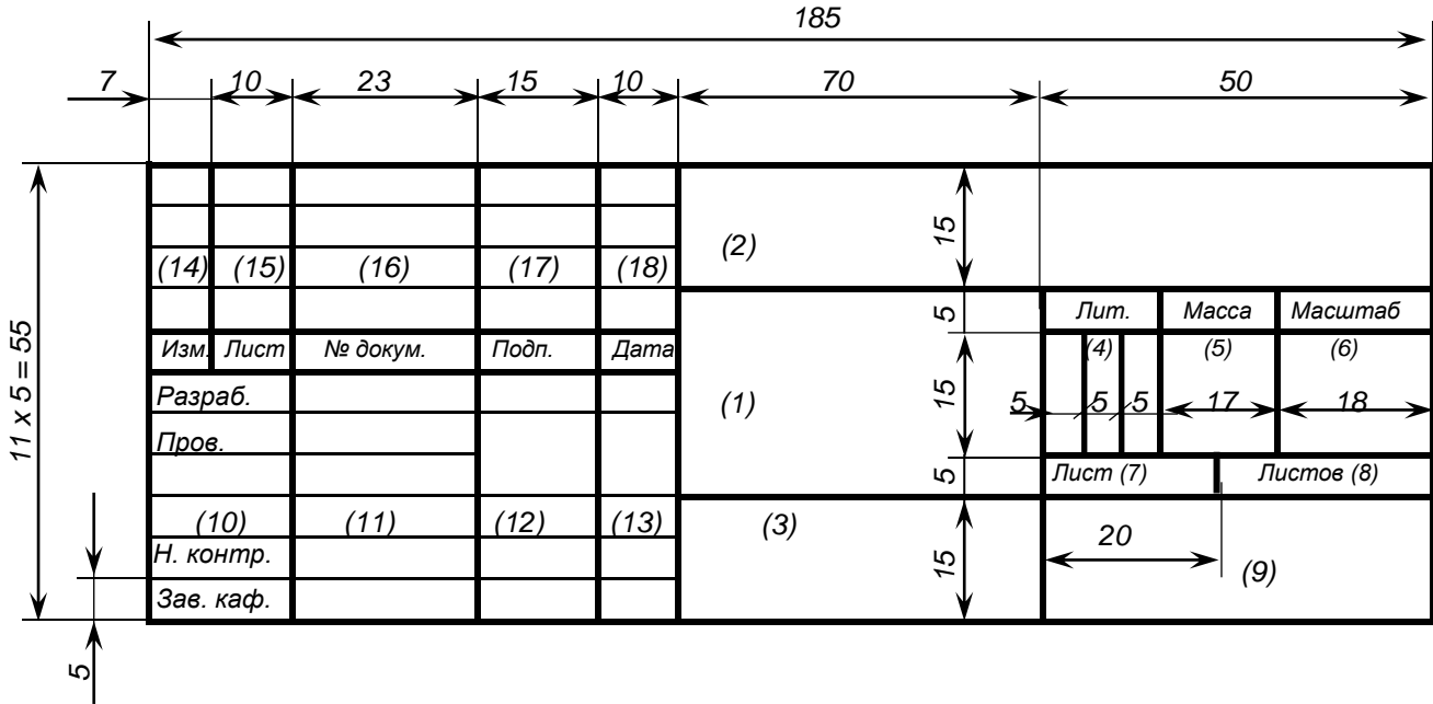
Рисунок Т.1 – Основная надпись для чертежей и схем (первый лист) по ГОСТ 2.104, форма 1
