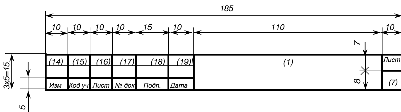
Рисунок Т.7 — Основная надпись и дополнительные графы к ней для чертежей строительных изделий и всех видов текстовых документов (последующие листы) по ГОСТ Р 21.1101, форма 6
