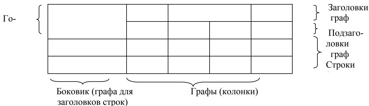
Рисунок 1 – Структура таблицы
