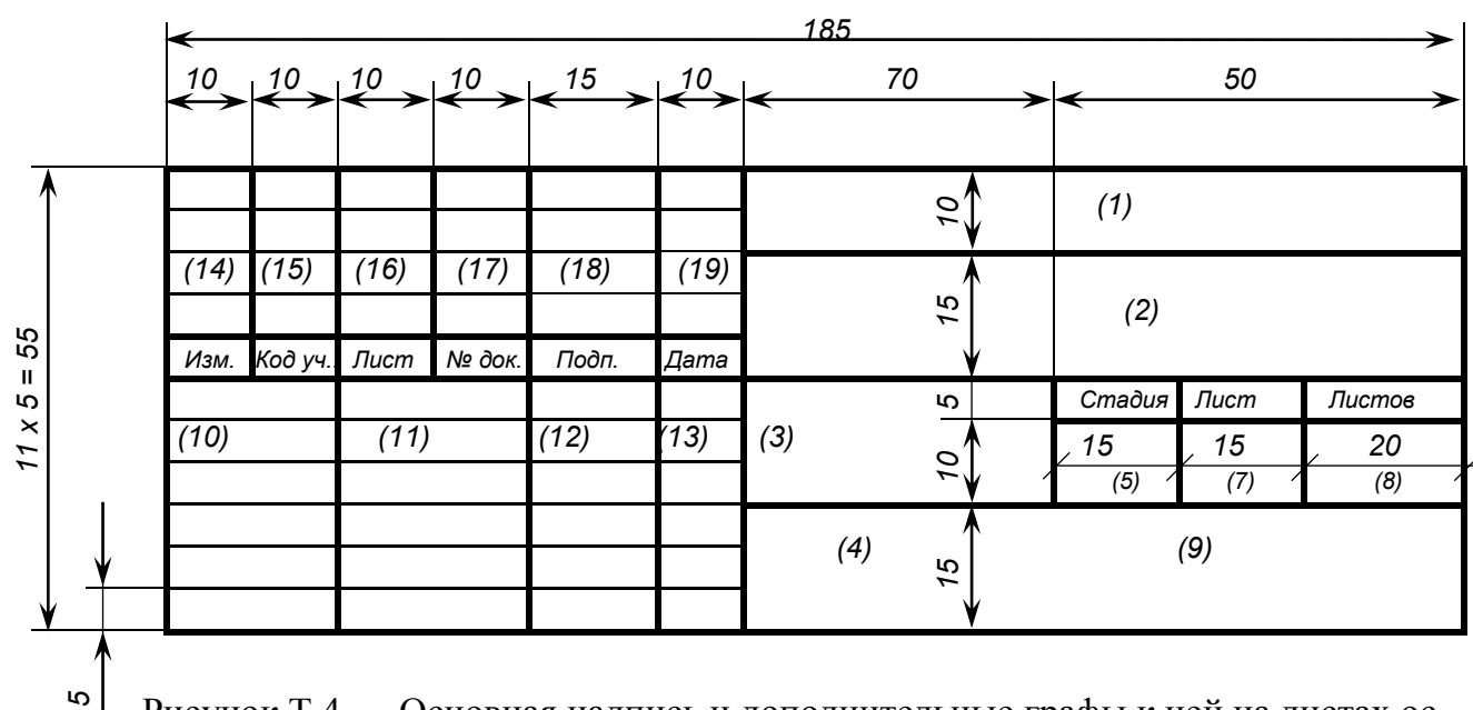
Рисунок Т.4 — Основная надпись и дополнительные графы к ней на листах основного комплекта рабочих чертежей по ГОСТ Р 21.1101, форма 3
