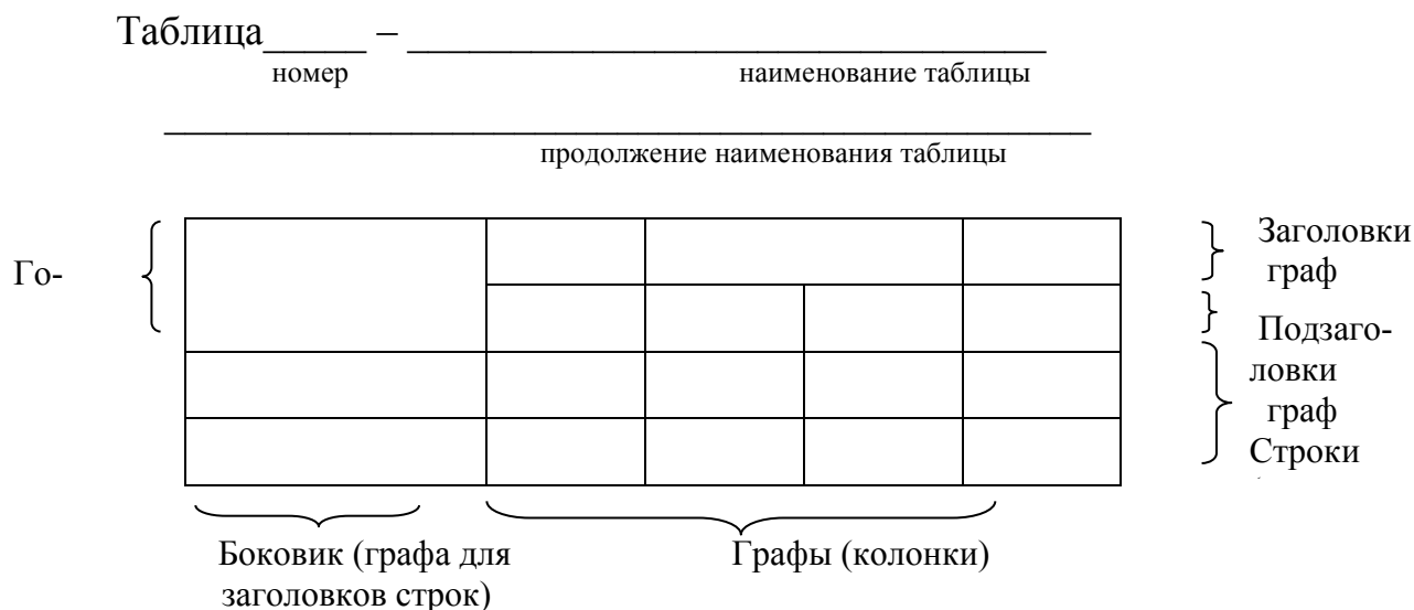
Рисунок 1 – Структура таблицы
